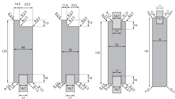
Riegel seitlich
