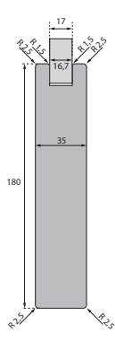
Sockel
