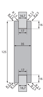
Querriegel
