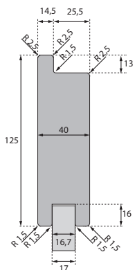
Riegel seitlich
