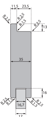
Riegel oben
